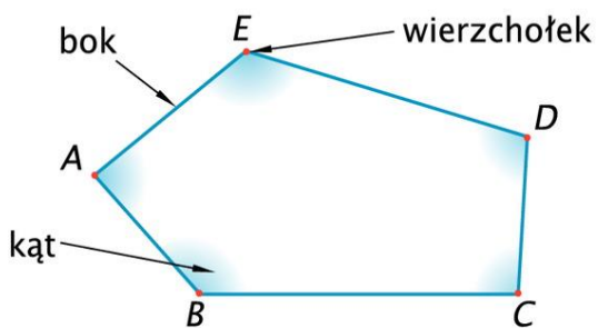
Pięciokąt ABCDE
